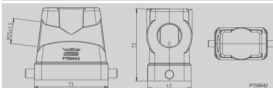
Tüllengehäuse Alu Höhe 72 mm mit Längsverriegelungsbügel Kabeleinführung seitlich
