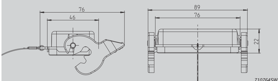
Schutzdeckel mit Längsverriegelungsbügel mit Dichtung und Fangschnur
