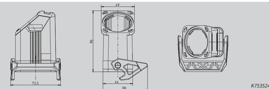
Kupplungsgehäuse Kunststoff Höhe 90 mm mit Längsverriegelungsbügel Kabeleinführung seitlich
