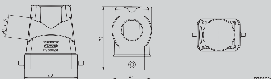
Tüllengehäuse Alu Höhe 72 mm mit Längsverriegelungsbügel Kabeleinführung seitlich
