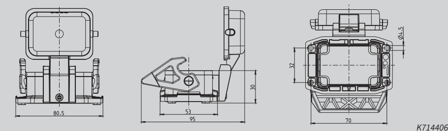
Anbaugehäuse Kunststoff Höhe 30 mm mit Längsverriegelungsbügel mit Klappdeckel
