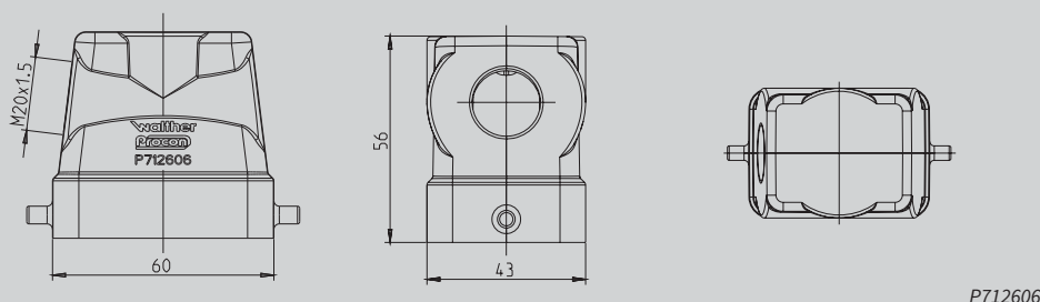
Tüllengehäuse Alu Höhe 56 mm mit Längsverriegelungsbügel Kabeleinführung seitlich
