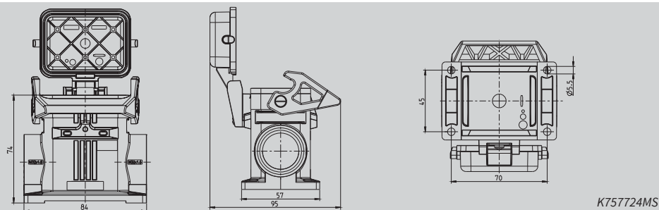
Sockelgehäuse Kunststoff Höhe 74 mm mit Längsverriegelungsbügel mit Klappdeckel
