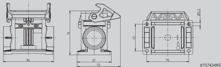
Sockelgehäuse Kunststoff Höhe 74 mm mit Längsverriegelungsbügel
