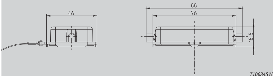
Schutzdeckel mit Fangschnur
