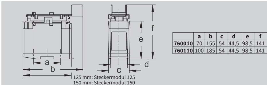
Steckermontageplatten, schwenkbar
