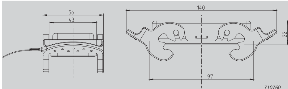
Schutzdeckel mit Dichtung und Fangschnur
