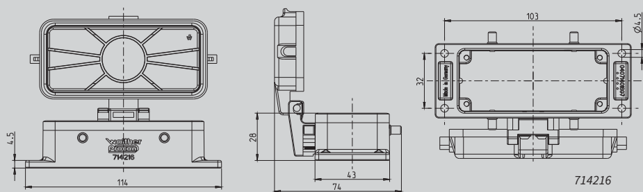
Anbaugehäuse Alu Höhe 28 mm für Querverriegelungsbügel mit Kunststoff-Klappdeckel
