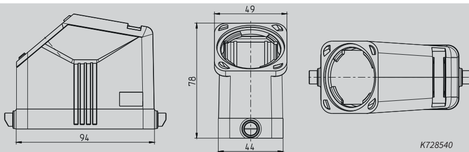
Tüllegehäuse Kunststoff Höhe 78 mm für Längsverriegelungsbügel Kabeleinführung seitlich
