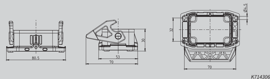
Anbaugehäuse Kunststoff Höhe 30 mm mit Längsverriegelungsbügel
